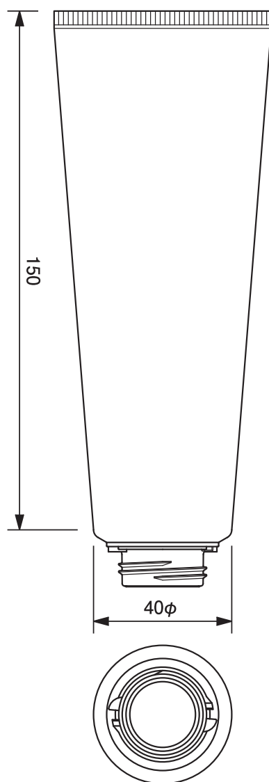
40φワンタッチチューブ -149.4 40mm dia. Flip-top Cap Tube-149.4
