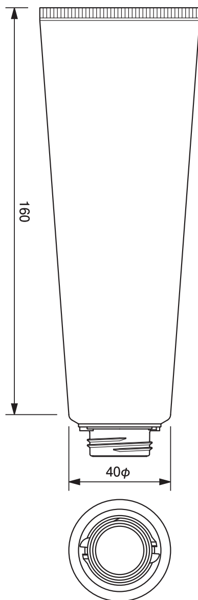
40φワンタッチチューブ -159.1 40mm dia. Flip-top Cap Tube-159.1
