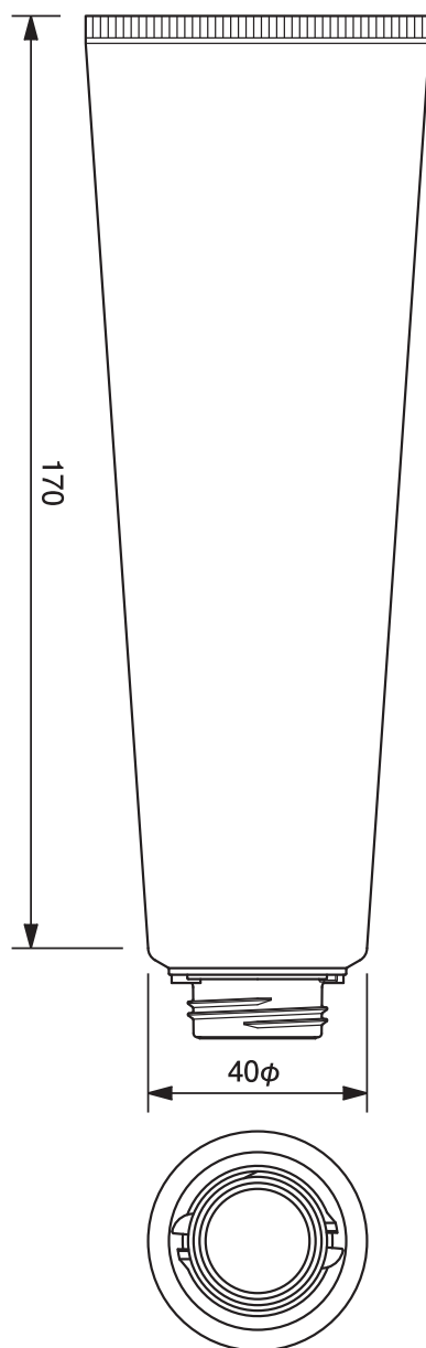
40φワンタッチチューブ -172.5 40mm dia. Flip-top Cap Tube-172.5
