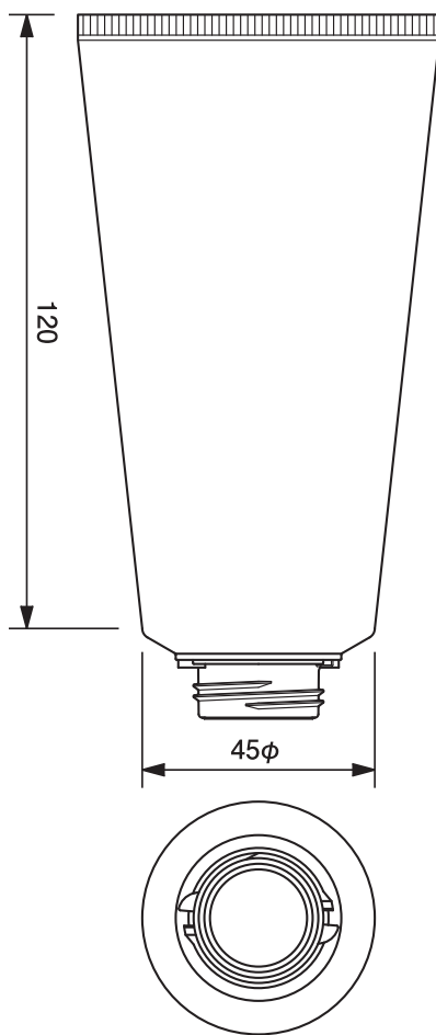
45φワンタッチチューブ -139.8 45mm dia. Flip-top Cap Tube-139.8
