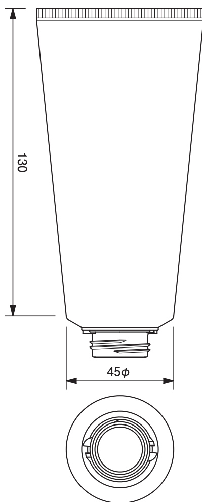
45φワンタッチチューブ -156.1 45mm dia. Flip-top Cap Tube-156.1
