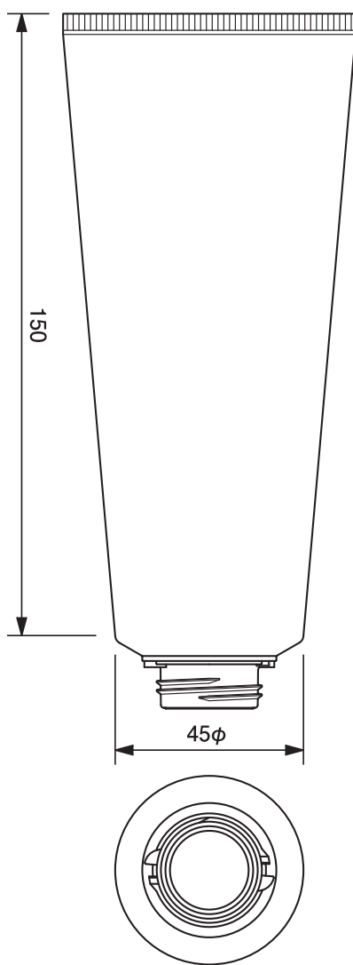
45φワンタッチチューブ -184.3 45mm dia. Flip-top Cap Tube-184.3
