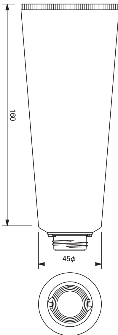
45φワンタッチチューブ -204.3 45mm dia. Flip-top Cap Tube-204.3
