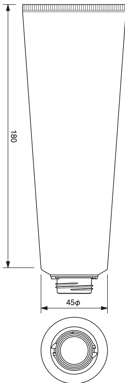
45φワンタッチチューブ -233.8 45mm dia. Flip-top Cap Tube-233.8
