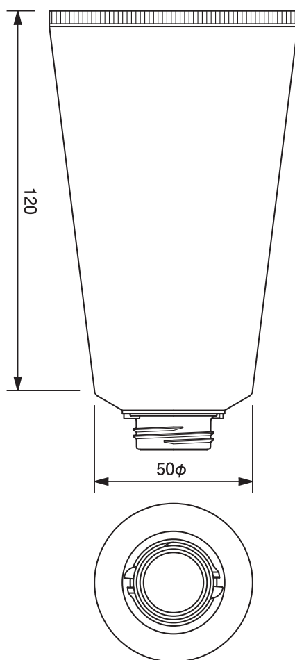
50φワンタッチチューブ -167.8 50mm dia. Flip-top Cap Tube-167.8
