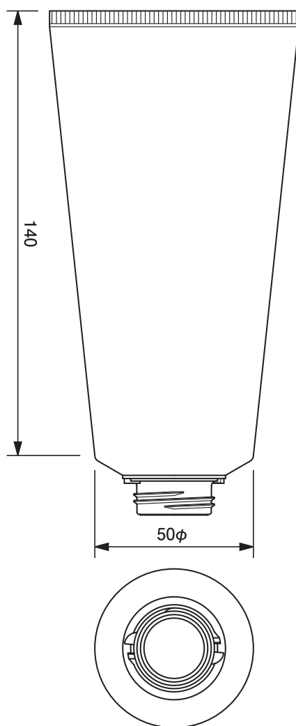
50φワンタッチチューブ -202.6 50mm dia. Flip-top Cap Tube-202.6
