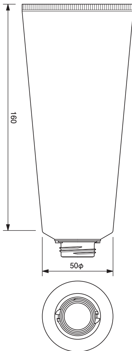
50φワンタッチチューブ -242.6 50mm dia. Flip-top Cap Tube-242.6
