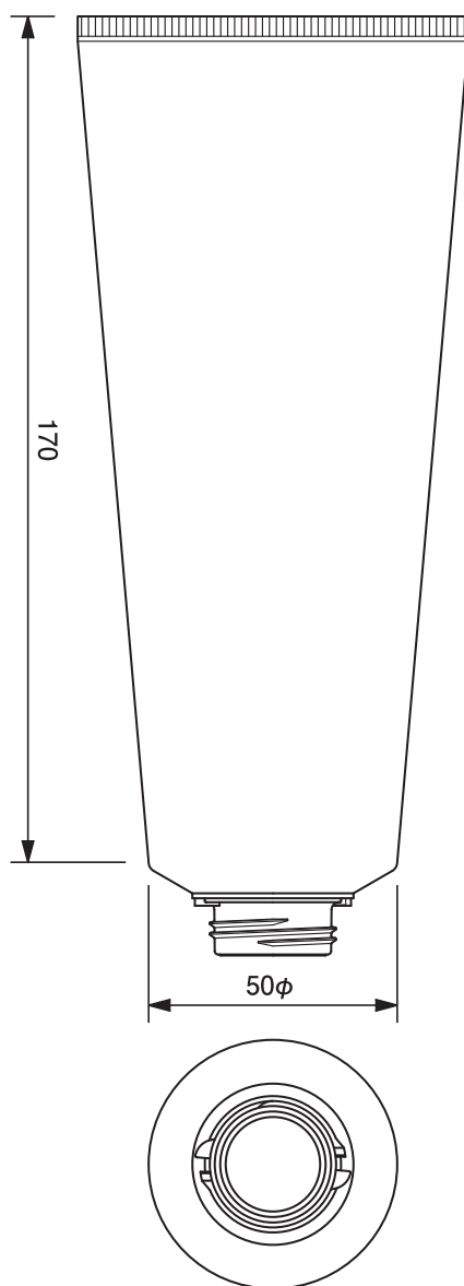
50φワンタッチチューブ -262.8 50mm dia. Flip-top Cap Tube-262.8
