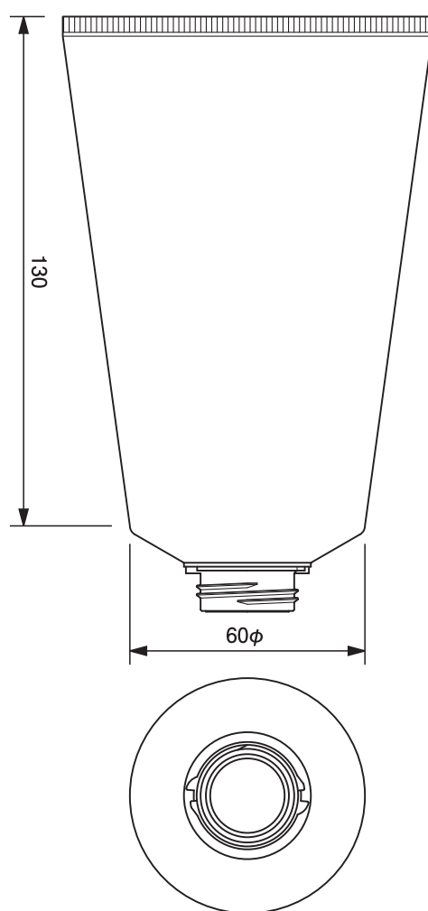
60φ共通チューブ -252.2 60mm dia. Tube-252.2
