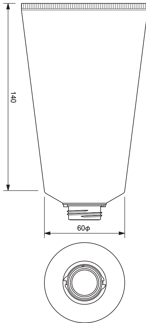
60φ共通チューブ -282.9 60mm dia. Tube-282.9
