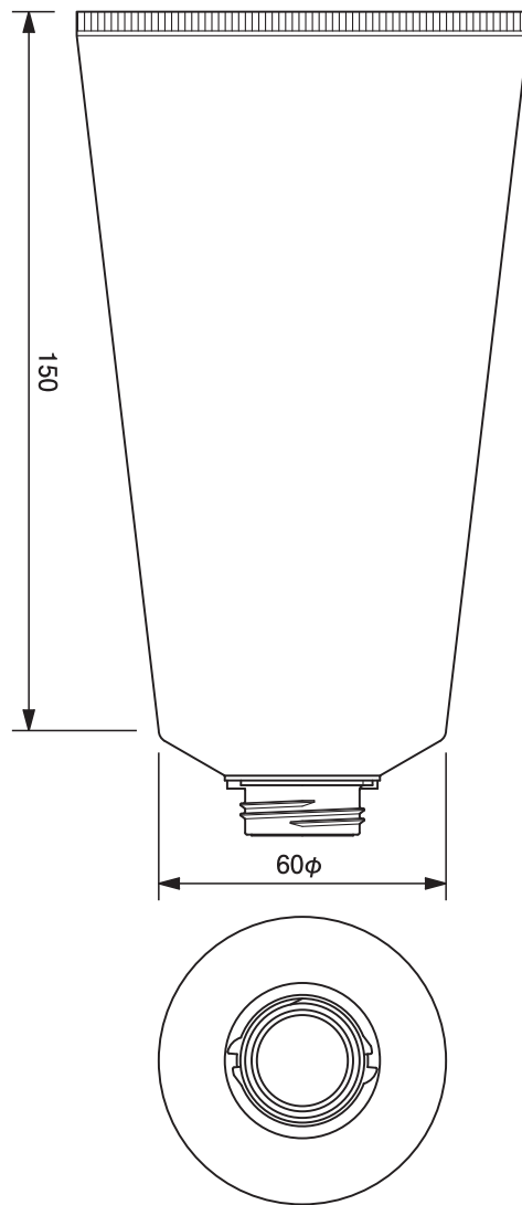
60φ共通チューブ -301.9 60mm dia. Tube-301.9
