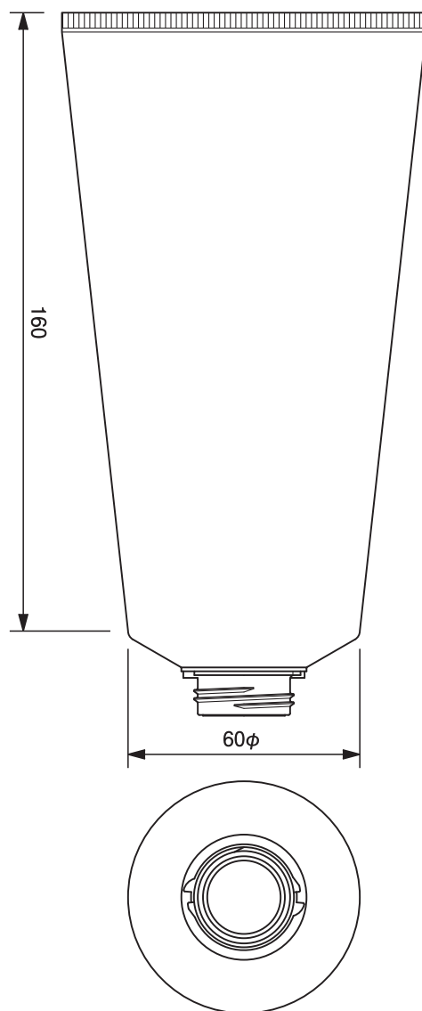
60φ共通チューブ -331.4 60mm dia. Tube-331.4
