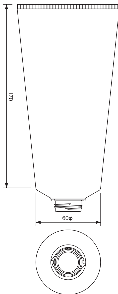
60φ共通チューブ -370.8 60mm dia. Tube-370.8
