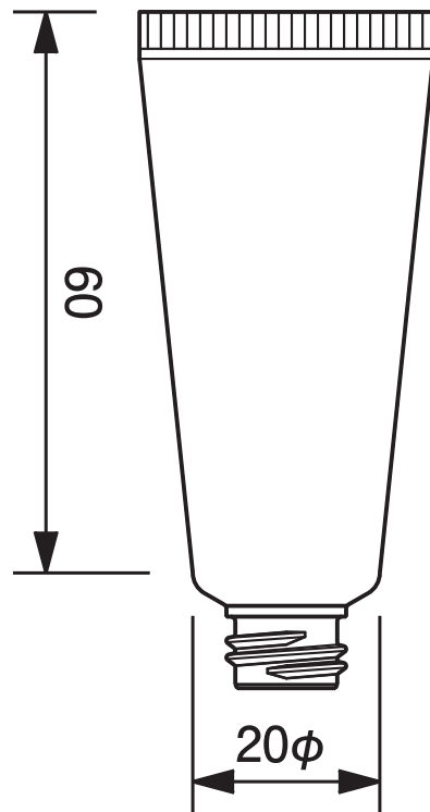
20φチューブ平ネジ用 -12.7 20mm dia. Tube-12.7
