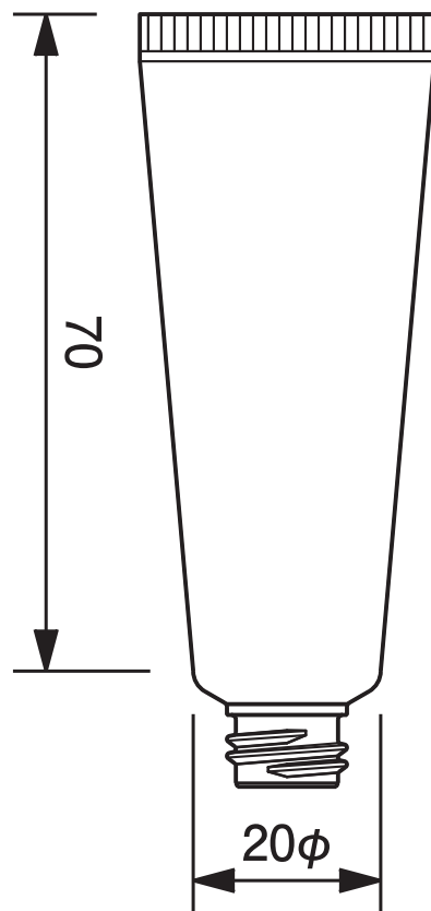
20φチューブ平ネジ用 -15.6 20mm dia. Tube-15.6
