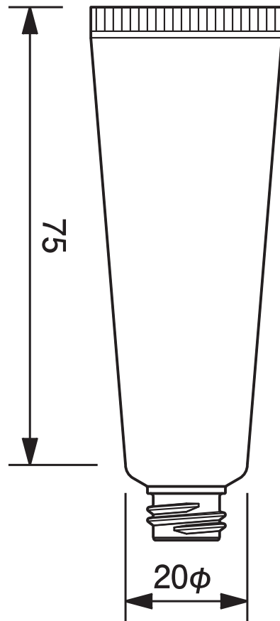
20φチューブ平ネジ用 -17.1 20mm dia. Tube-17.1
