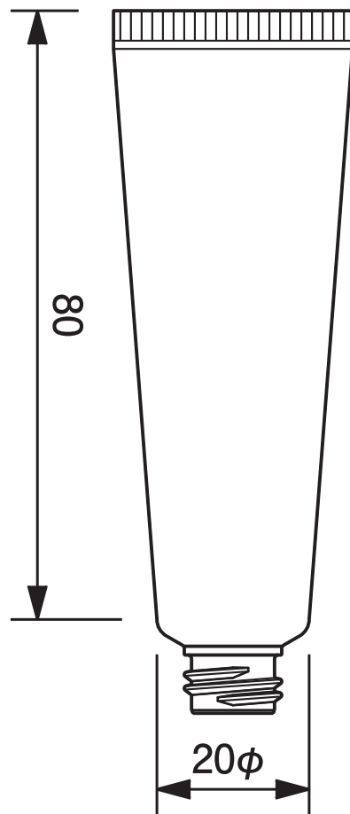
20φチューブ平ネジ用 -18.5 20mm dia. Tube-18.5
