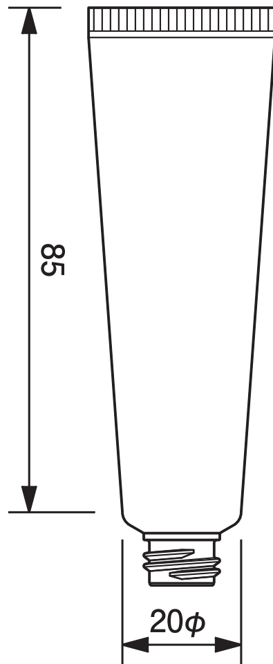
20φチューブ平ネジ用 -19.8 20mm dia. Tube-19.8
