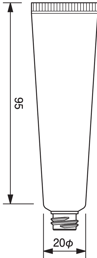
20φチューブ平ネジ用 -22.8 20mm dia. Tube-22.8
