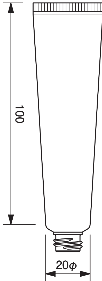
20φチューブ平ネジ用 -24.3 20mm dia. Tube-24.3
