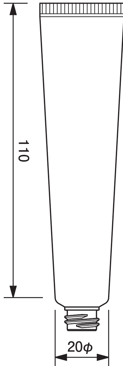
20φチューブ平ネジ用 -27.4 20mm dia. Tube-27.4
