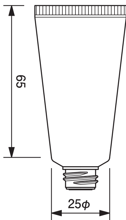
25φチューブ平ネジ用 -21.1 25mm dia. Tube-21.1
