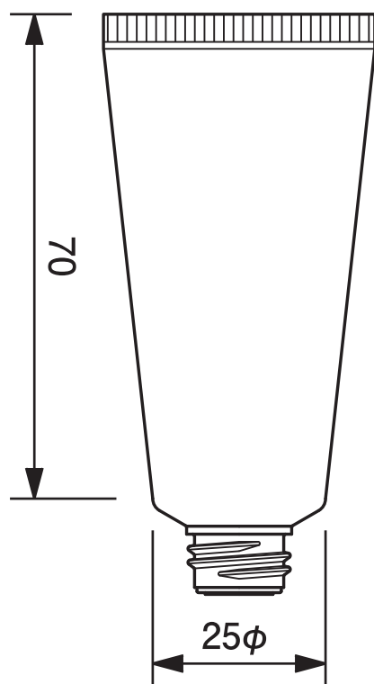
25φチューブ平ネジ用 -23.6 25mm dia. Tube-23.6
