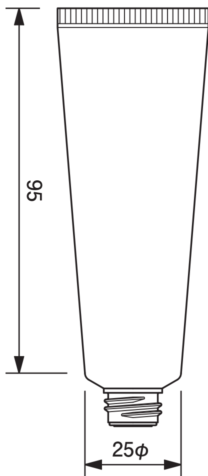
25φチューブ平ネジ用 -35.2 25mm dia. Tube-35.2
