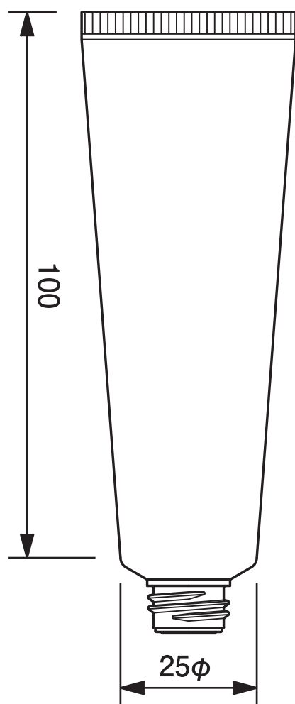
25φチューブ平ネジ用 -37.7 25mm dia. Tube-37.7
