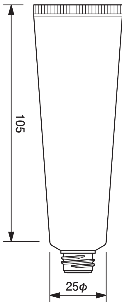
25φチューブ平ネジ用 -39.7 25mm dia. Tube-39.7
