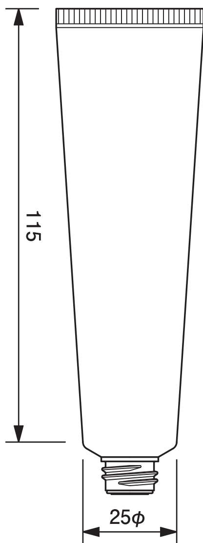
25φチューブ平ネジ用 -45.4 25mm dia. Tube-45.4
