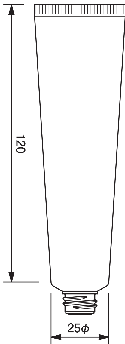
25φチューブ平ネジ用 -47.2 25mm dia. Tube-47.2
