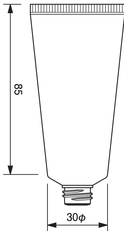
30φチューブ平ネジ用 -42.5 30mm dia. Tube-42.5
