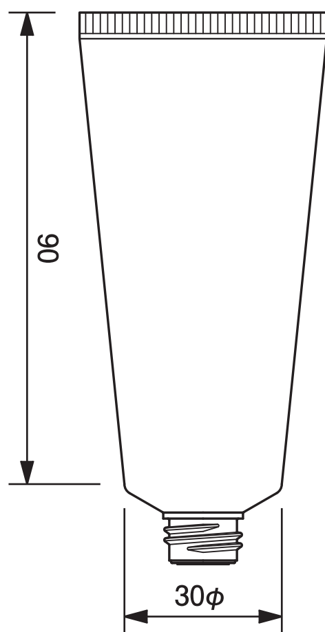
30φチューブ平ネジ用 -44.8 30mm dia. Tube-44.8
