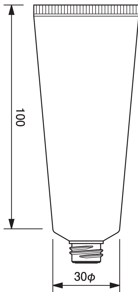
30φチューブ平ネジ用 -51.8 30mm dia. Tube-51.8
