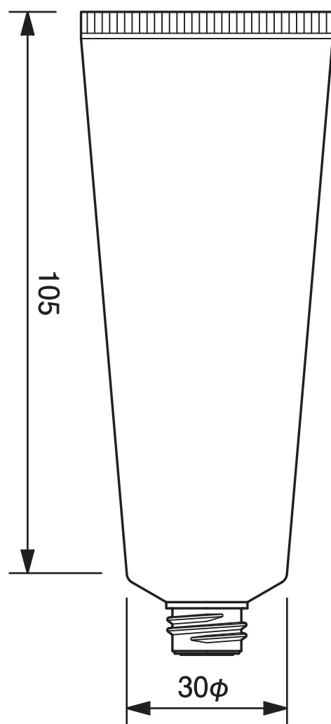
30φチューブ平ネジ用 -54.6 30mm dia. Tube-54.6
