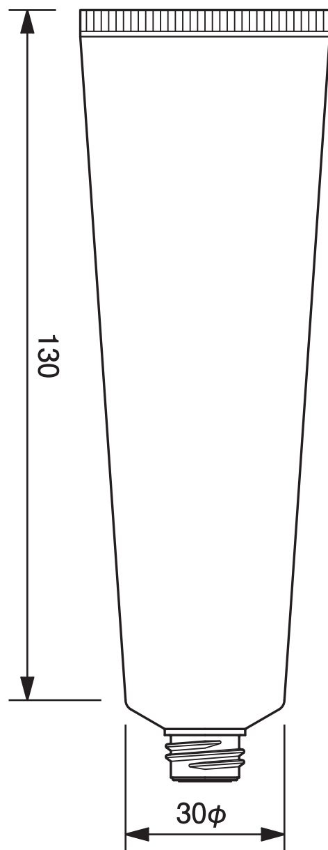
30φチューブ平ネジ用 -71.8 30mm dia. Tube-71.8
