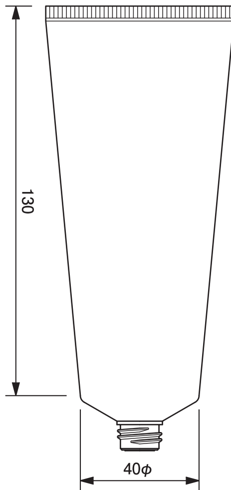
40φチューブ平ネジ用 -124.6 40mm dia. Tube-124.6
