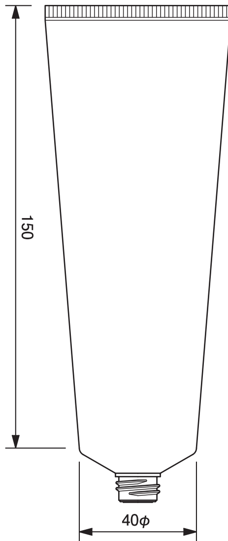
40φチューブ平ネジ用 -149.4 40mm dia. Tube-149.4
