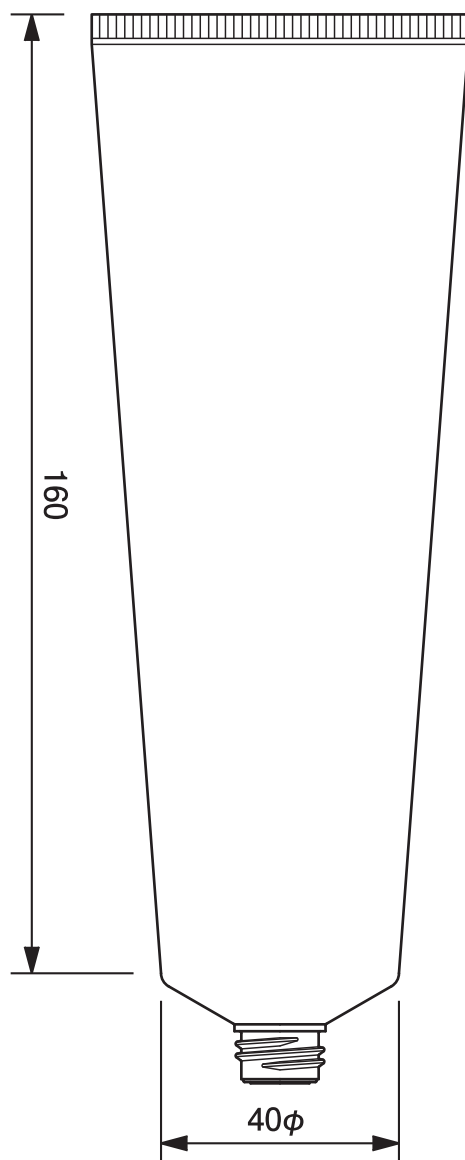
40φチューブ平ネジ用 -159.1 40mm dia. Tube-159.1
