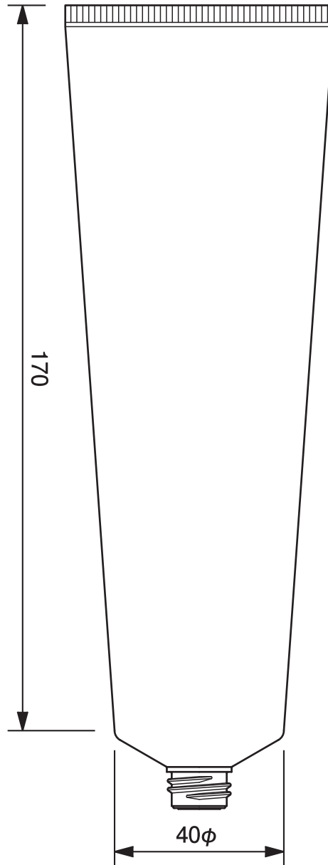
40φチューブ平ネジ用 -172.5 40mm dia. Tube-172.5
