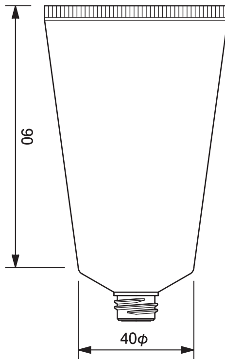
40φチューブ平ネジ用 -78.3 40mm dia. Tube-78.3
