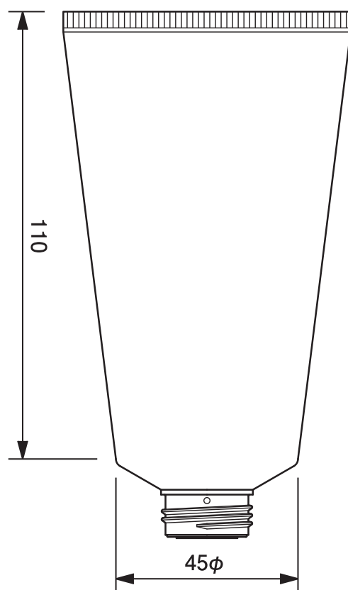
45φチューブ平ネジ用 -125.5 45mm dia. Tube-125.5
