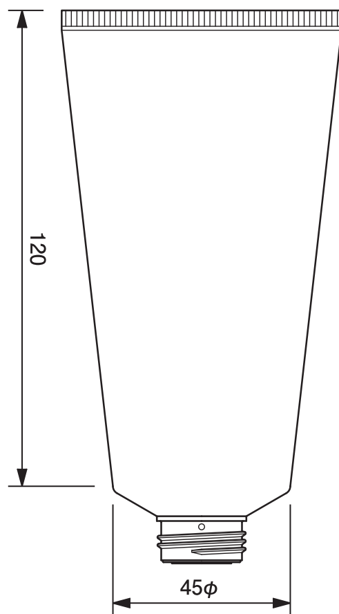
45φチューブ平ネジ用 -139.8 45mm dia. Tube-139.8
