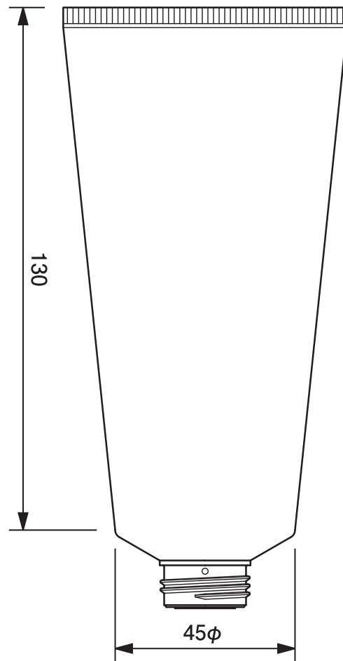
45φチューブ平ネジ用 -156.1 45mm dia. Tube-156.1
