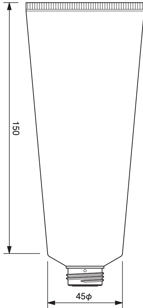
45φチューブ平ネジ用 -184.3 45mm dia. Tube-184.3
