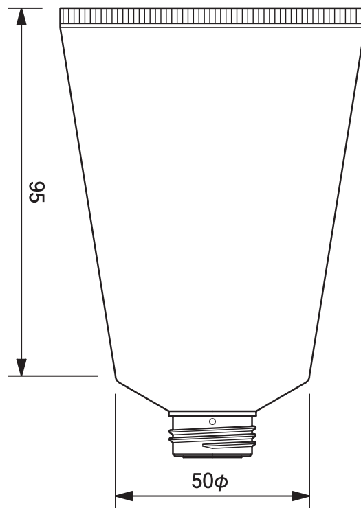
50φチューブ平ネジ用 -124.2 50mm dia. Tube-124.2
