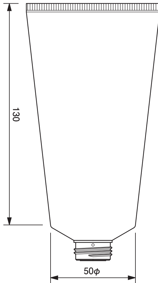
50φチューブ平ネジ用 -181.9 50mm dia. Tube-181.9
