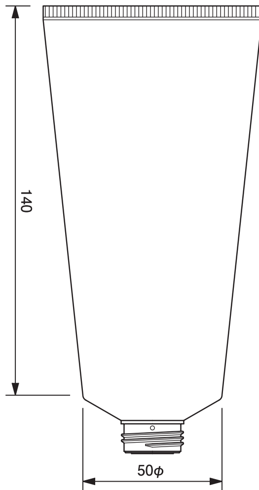
50φチューブ平ネジ用 -202.6 50mm dia. Tube-202.6
