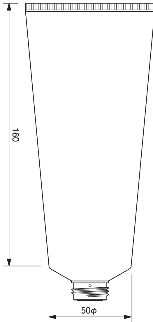
50φチューブ平ネジ用 -242.6 50mm dia. Tube-242.6
